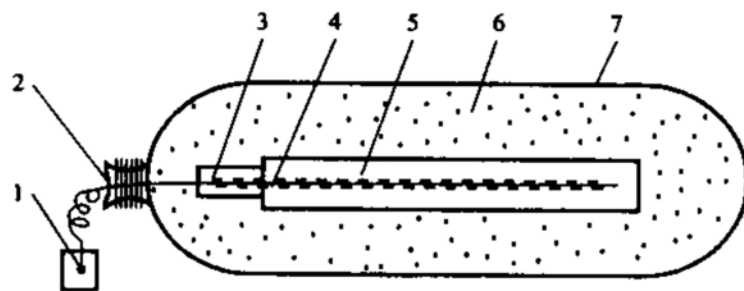
图 C.9 埋地阳极组装示意图
